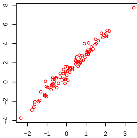
Dépendance linéaire positive
