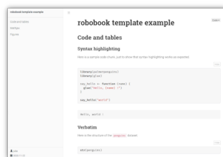
Figure 13.18.: Modèle robobook
