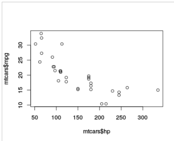
Figure 13.3.: Rendu docx
