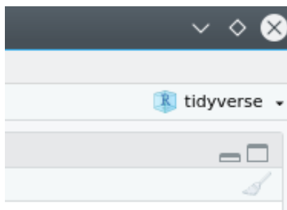
Figure 5.2.: Menu projets
