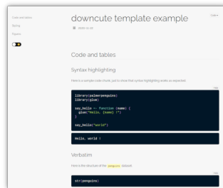
Figure 13.17.: Modèle downcute
