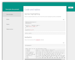
Figure 13.19.: Modèle material
