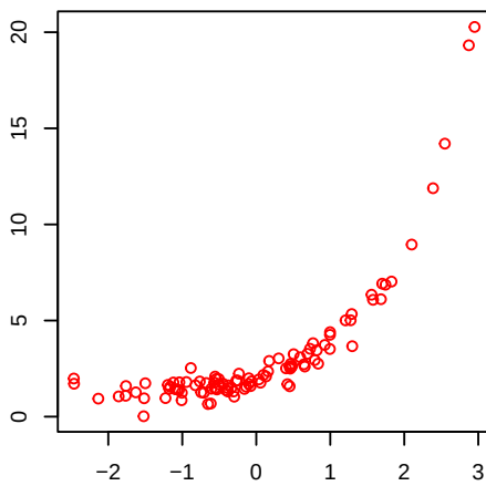
Dépendance non-linéaire monotone
