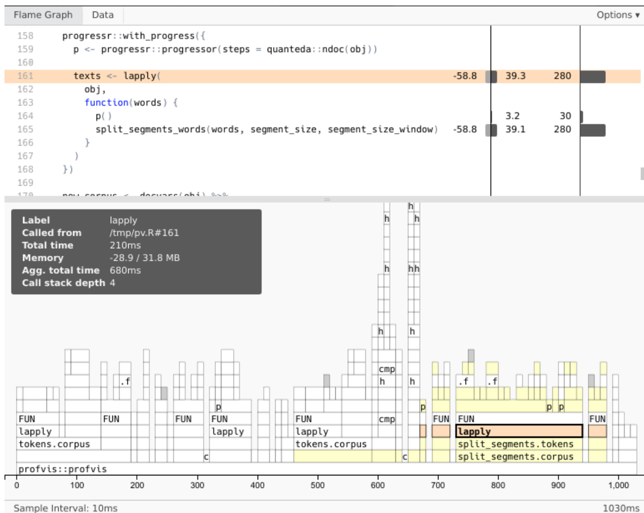
Figure 20.1.: Exemple de visualisation générée par profvis()
